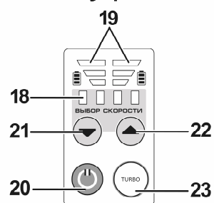
Панель управления
