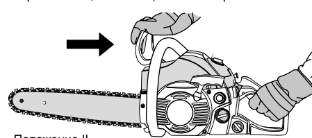
Положение II. Тормоз не нажат, пильная цепь не заблокирована.
