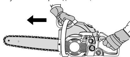
Положение I. Тормоз нажат, пильная цепь заблокирована.
