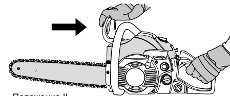
Положение II. Тормоз не нажат, пильная цепь не заблокирована.
